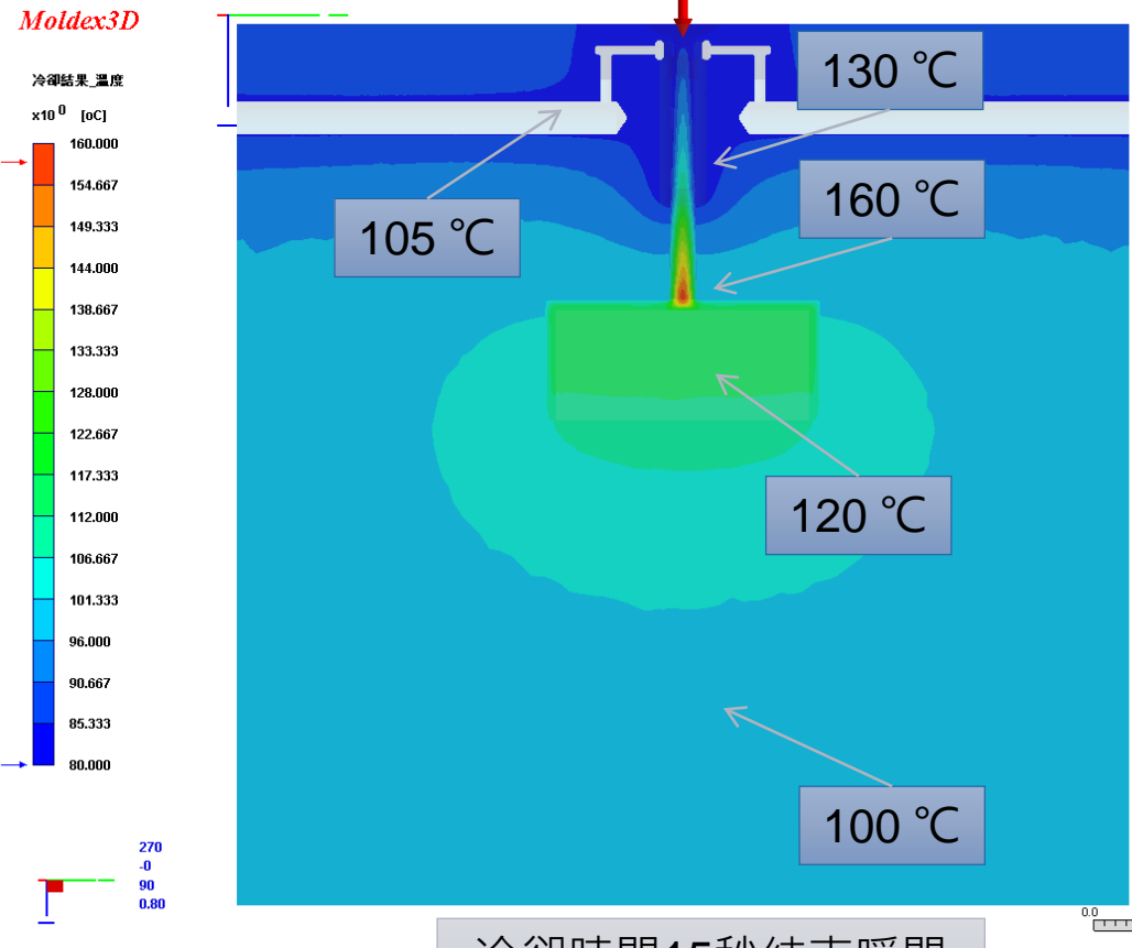
冷卻時間15秒結束瞬間 模具溫度分佈
